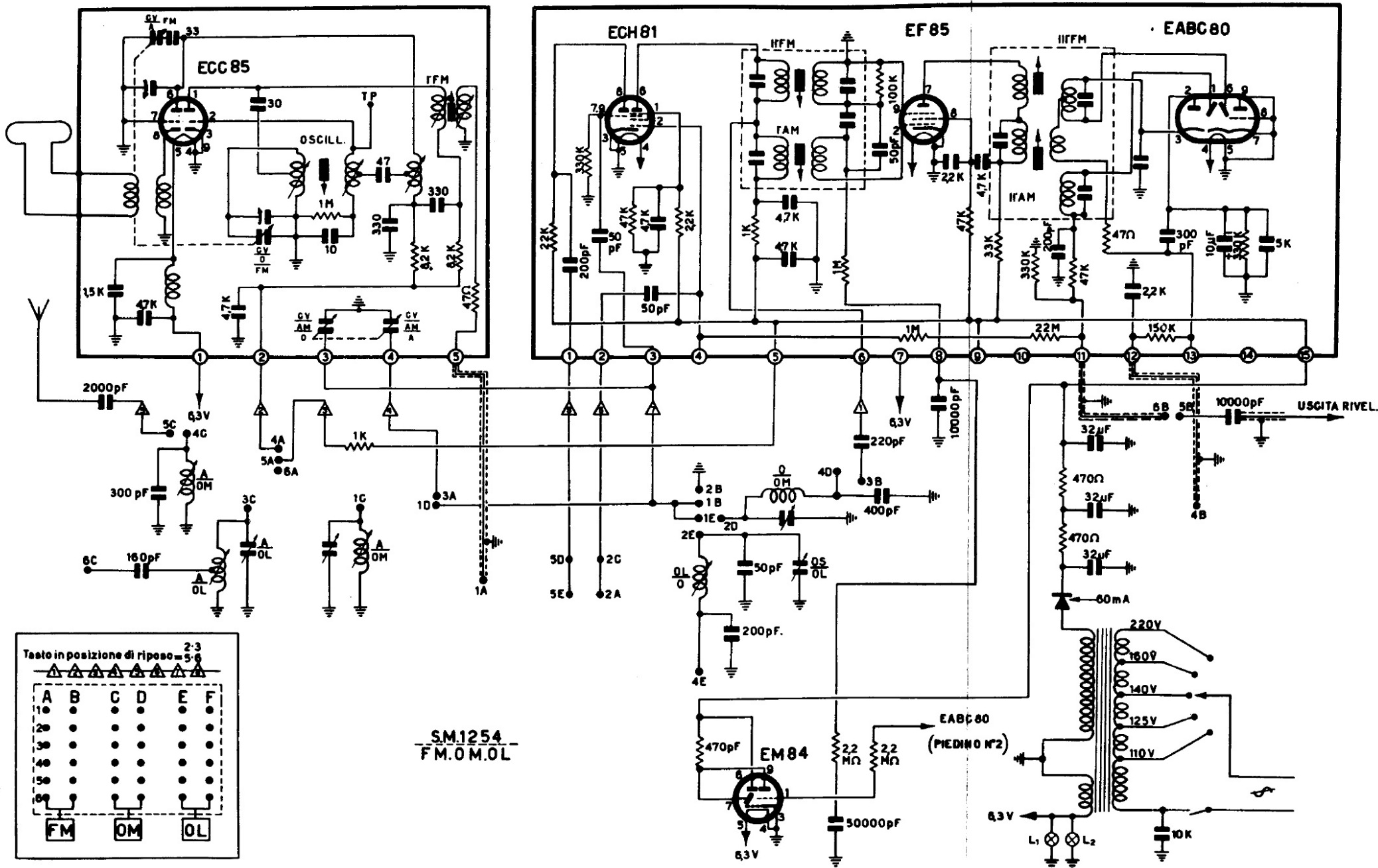
CASTELFRANCHI G.B. - Mod. SM 1254. Sintonizzatore per funzionare con amplificatore ad alta fedeltà. È a modulazione di ampiezza e di frequenza, e consente la ricezione delle emittenti ad onde lunghe, medie e ultracorte, essendo provvisto di selettore di produzione tedesca. È fornito in scatola di montaggio.
